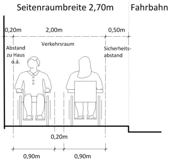
Abbildung 94: Skizze des Raumbedarfs für die Begegnung zweier Rollstühle
